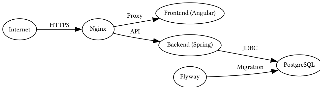
Fig. 11. – Architecture physique et logique de l'infrastructure PIAWEB
