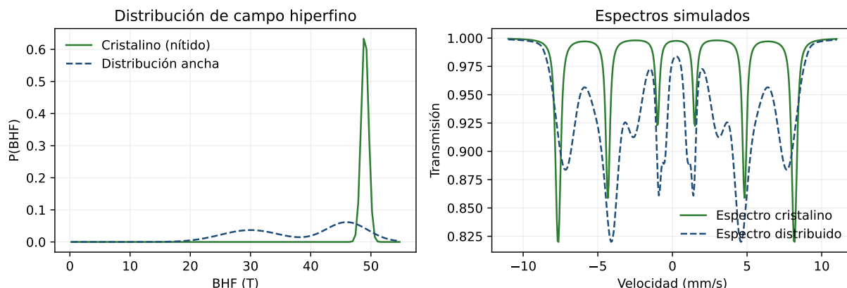
Figura 5.1: Izquierda: distribución de campo hiperfino cristalina (nítida, en torno a 49 T) frente a una distribución ancha. Derecha: los espectros simulados correspondientes. La distribución ancha «emborrona» y solapa las líneas del sexteto.
