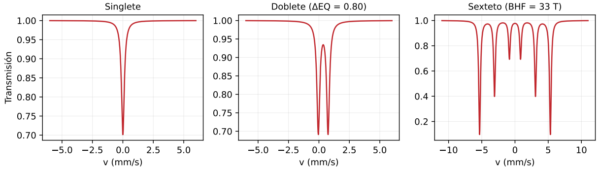
Figura 4.1: Simulación de los tres componentes discretos: singlete (un pico), doblete ( \Delta E_Q = 0,80 mm/s) y sexteto ( B_{\text{hf}} = 33 T con relación de intensidades 3 : 2 : 1).
