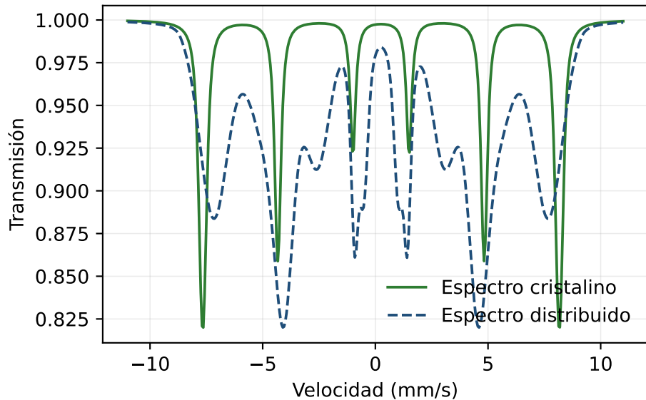
Espectros simulados
