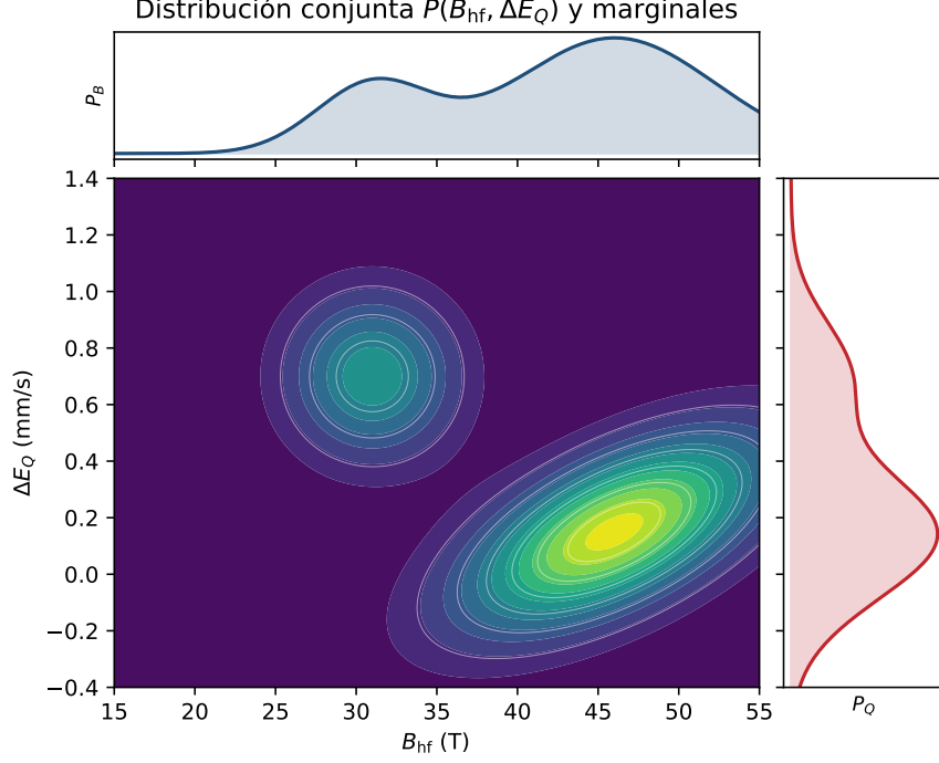
Figura 1: Distribución conjunta P(B_{\text{hf}}, \Delta E_Q) y sus marginales. El mapa central muestra dos poblaciones: una nube inclinada (campo alto, cuadrupolo pequeño), cuya inclinación indica correlación aparente \rho_{BQ} , y un segundo sitio aislado. Arriba y a la derecha, las marginales P_B y P_Q obtenidas integrando el mapa; por sí solas no revelan la correlación, que sólo se ve en el mapa 2D.
