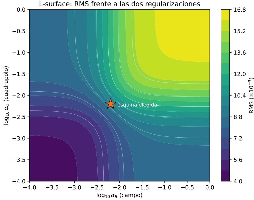
Figura 2: L-surface de regularización 2D, análoga a la L-curve pero con dos parámetros. El RMS es bajo cuando ambas regularizaciones son débiles (esquina inferior izquierda: el mapa ajusta el ruido) y crece al reforzarlas (arriba a la derecha: sobre-suavizado). La esquina de compromiso (estrella) equilibra ajuste y suavidad en cada eje; conviene comprobar que la solución es estable alrededor de ella.
