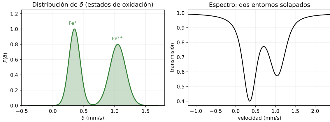
Figura 1: Distribución de desplazamiento isomérico. Izquierda : una P(\delta) con dos poblaciones separadas en \delta —por ejemplo \text{Fe}^{3+} ( \delta \approx 0,35 mm/s) y \text{Fe}^{2+} ( \delta \approx 1,05 mm/s)— refleja dos estados de oxidación o entornos. Derecha : el espectro resultante es la superposición de los patrones de cada \delta ; cuando los entornos solapan, la información los separa mejor que un ajuste discreto rígido.
