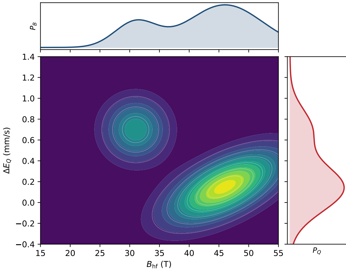
Distribución conjunta P(B_{\text{hf}}, \Delta E_Q) y marginales
