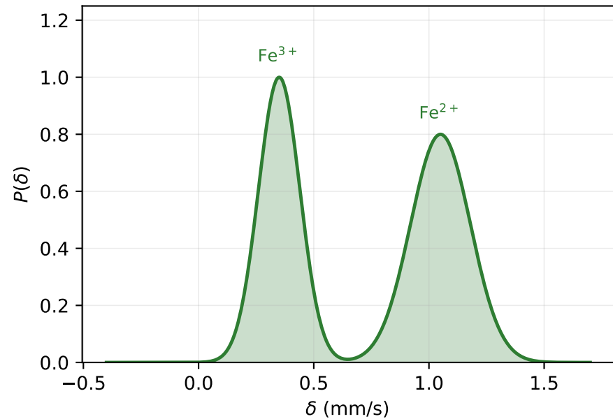
Distribución de \delta (estados de oxidación)
