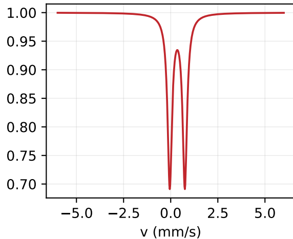
Doblete ( \Delta EQ = 0.80 )
