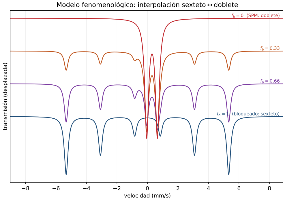
Figura D.1: Modelo fenomenológico Relajacion (D.5). Al bajar la fracción bloqueada f_b de 1 (sexteto bloqueado) a 0 (doblete superparamagnético aparente), la señal del sexteto se transfiere a un doblete central de área equivalente. No representa dos fases químicas, sino el efecto espectral de la relajación.
