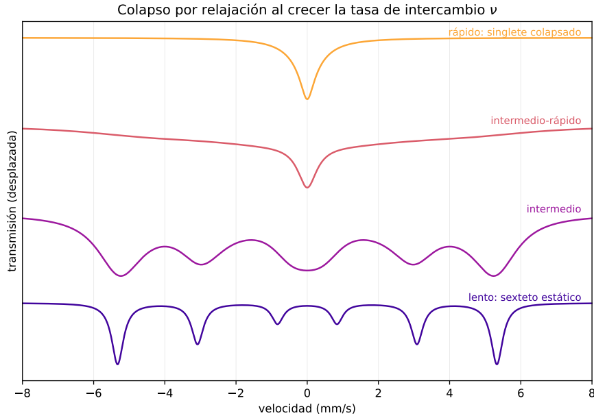
Figura D.2: Colapso por relajación en el modelo de dos estados +B_{\text{hf}} \leftrightarrow -B_{\text{hf}} (D.15). A tasa baja (abajo) el espectro es el sexteto estático ; al crecer la tasa las líneas se ensanchan y coalescen ( régimen intermedio ); a tasa alta (arriba) las posiciones magnéticas se promedian a cero y queda una única línea colapsada . Curvas desplazadas verticalmente para comparar.
