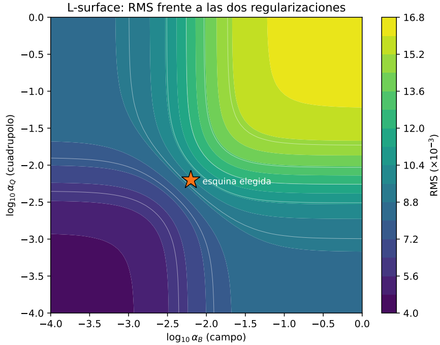
Figura C.2: L-surface de regularización 2D, análoga a la L-curve pero con dos parámetros. El RMS es bajo cuando ambas regularizaciones son débiles (esquina inferior izquierda: el mapa ajusta el ruido) y crece al reforzarlas (arriba a la derecha: sobre-suavizado). La esquina de compromiso (estrella) equilibra ajuste y suavidad en cada eje; conviene comprobar que la solución es estable alrededor de ella.
