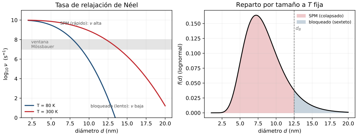
Figura D.3: Néel–Arrhenius: bloqueo por tamaño. Izquierda : la tasa de relajación \nu(d, T) cae al crecer el diámetro; las partículas pequeñas relajan rápido (superparamagnéticas, colapsan a singlete/doblete) y las grandes quedan bloqueadas (sexteto). Una partícula se ve bloqueada cuando \nu baja de la ventana de observación Mössbauer (banda gris); al bajar T el bloqueo se desplaza a diámetros menores. Derecha : sobre una distribución lognormal de tamaños, a T fija el diámetro de bloqueo d_B separa la fracción superparamagnética de la bloqueada, y el espectro es la mezcla de ambas.
