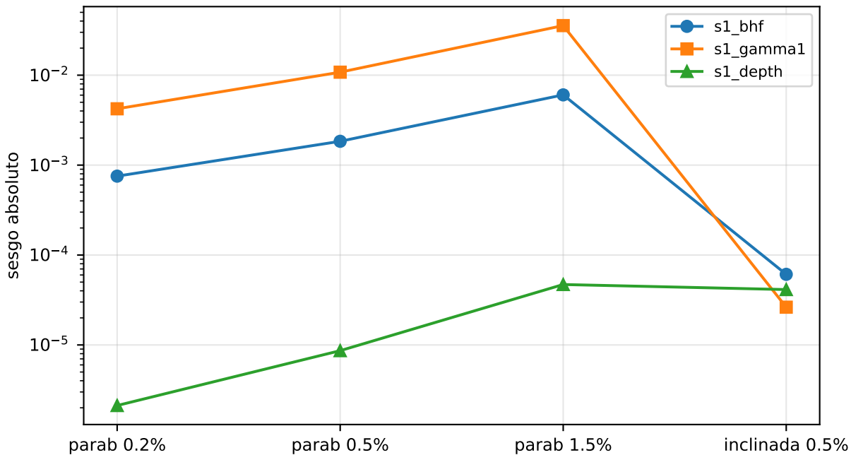
E3 — base no plana: sesgo con el modelo baseline+slope de Fitbauer (sin término de curvatura)
