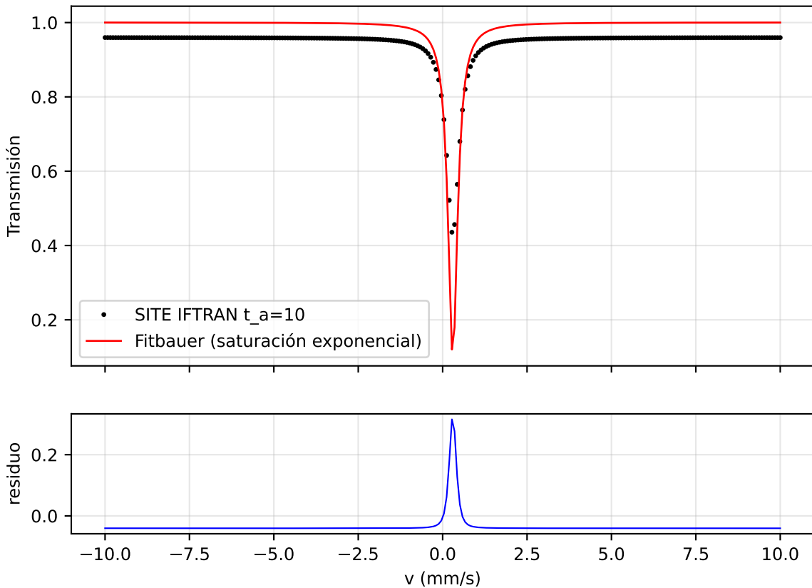
F1_t10 — forma de línea de transmisión gruesa
