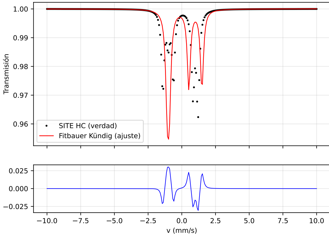
A4_R2_th90 — SITE recalcula intensidades y transiciones \Delta m_l = \pm 2 ; el Kündig de Fitbauer solo mueve posiciones
