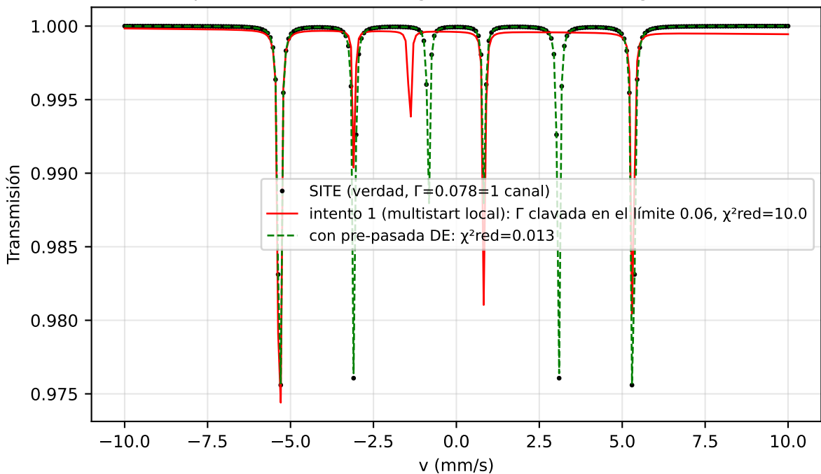
C4 — \Gamma \approx anchura de canal: cuenca de convergencia \sim \Gamma (con arranque exacto o DE el sesgo es < 4e-4 T: convergencia, no modelo)
