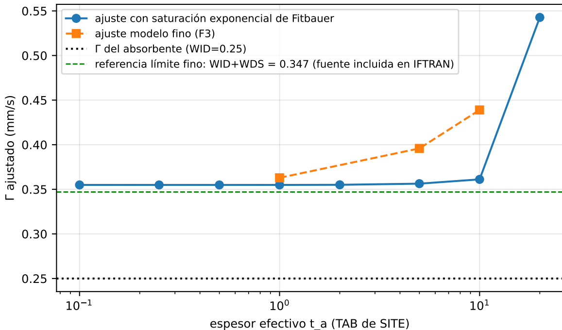
F — integral de transmisión de SITE vs modelos de Fitbauer: el ensanchamiento por espesor no es capturado por la saturación exponencial
