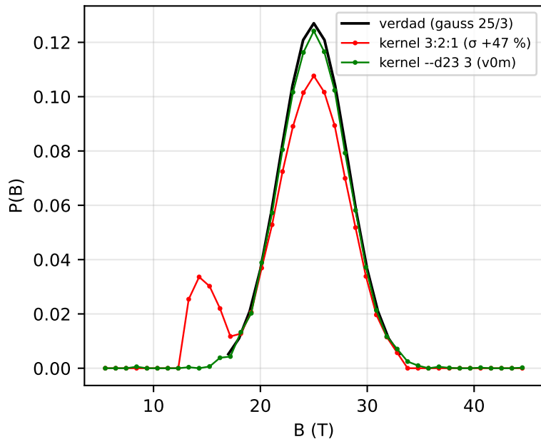
L6 — textura D23=3 de DIST: el kernel clásico deforma P(B)
