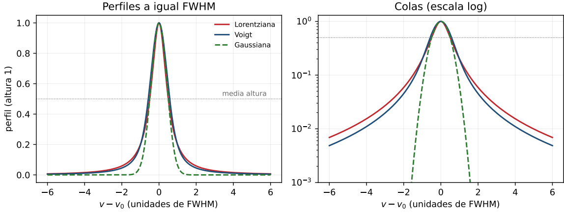
Figura A.1: Perfiles de línea normalizados a altura unidad y a igual FWHM. La Lorentziana (A.3) tiene colas pesadas ; la Gaussiana decae mucho más deprisa; el pseudo-Voigt (A.5) interpola entre ambas. La escala logarítmica (derecha) hace visible el peso de las colas, que es lo que distingue a un perfil de otro lejos del centro.
