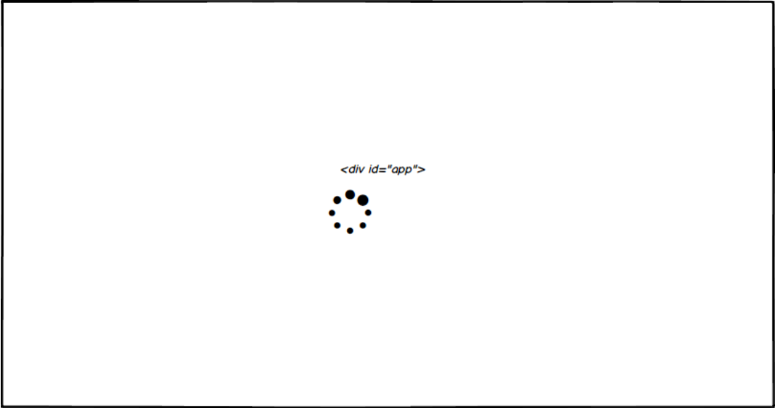
App.razor
