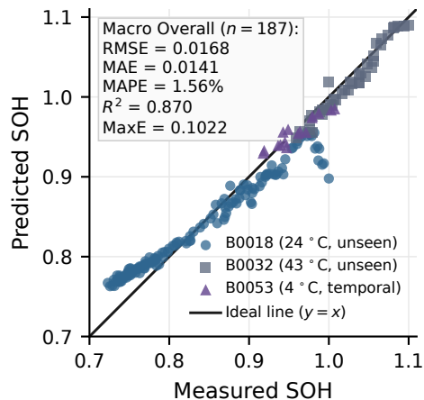
(d) Parity plot (All 187 test cycles)
