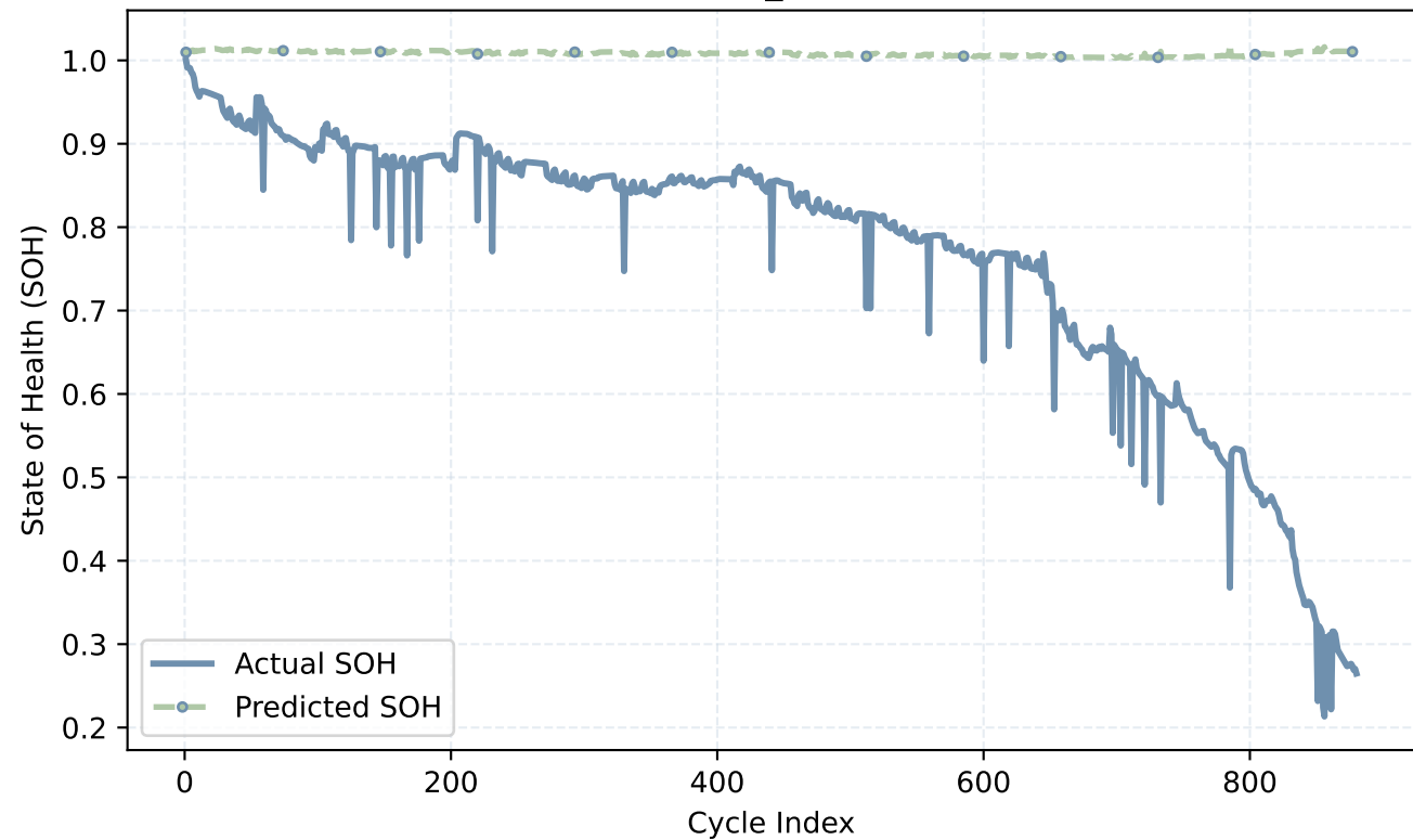
NASA→CALCE zero-shot CS2_35: Actual vs Predicted SOH
