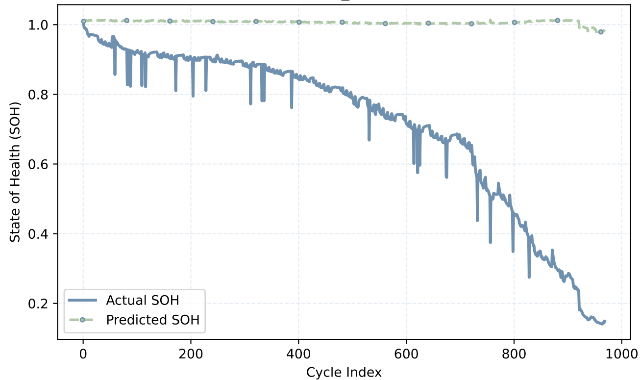
NASA→CALCE zero-shot CS2_36: Actual vs Predicted SOH
