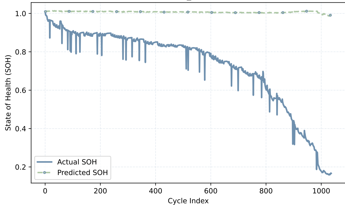
NASA→CALCE zero-shot CS2_37: Actual vs Predicted SOH
