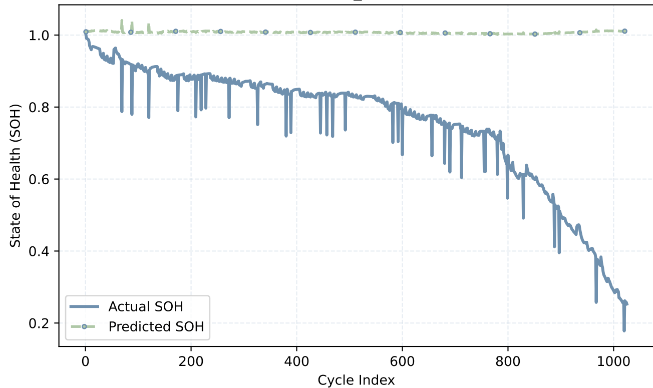
NASA→CALCE zero-shot CS2_38: Actual vs Predicted SOH
