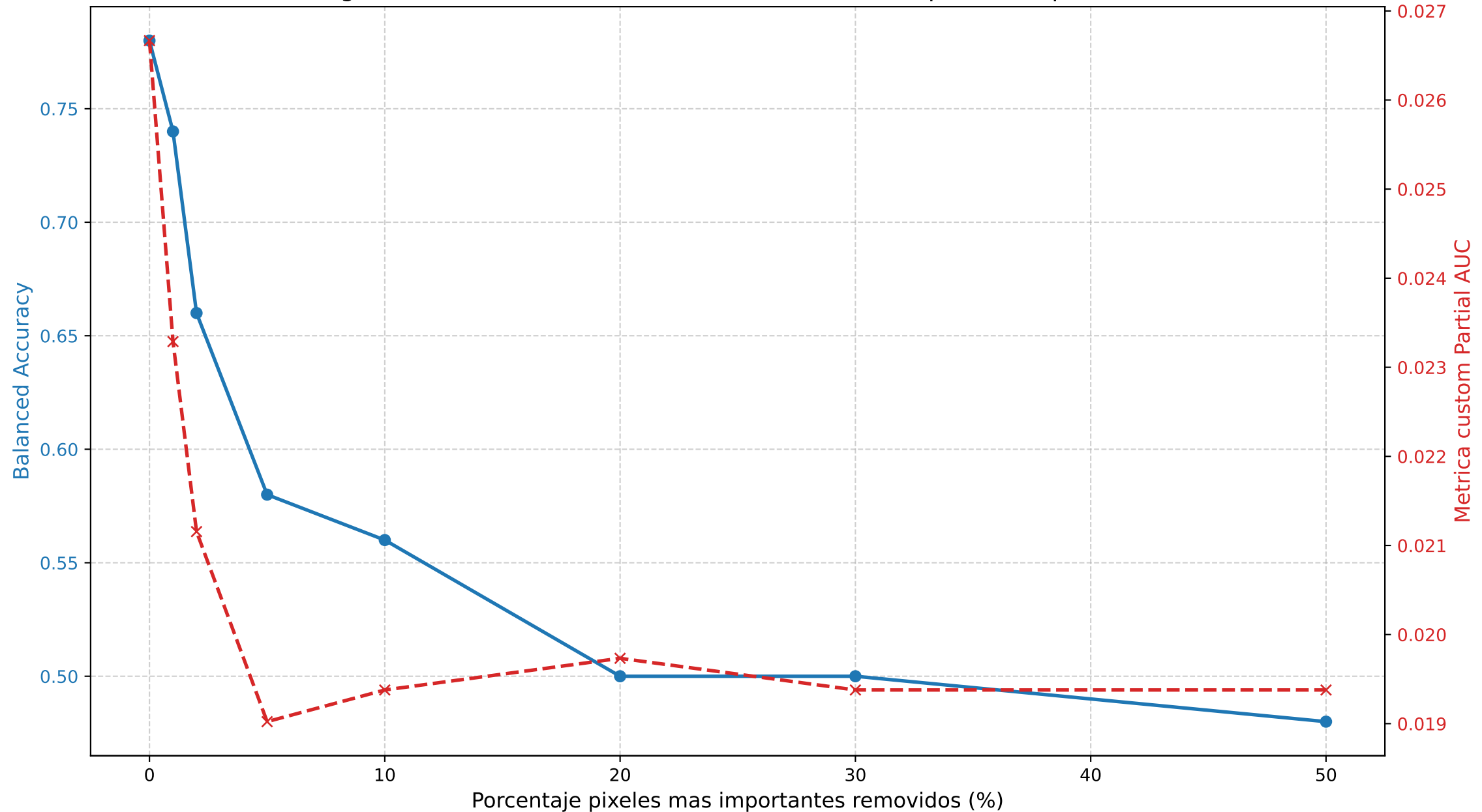
Degradación rendimiento modelo vs. Perturbación pixeles importantes
