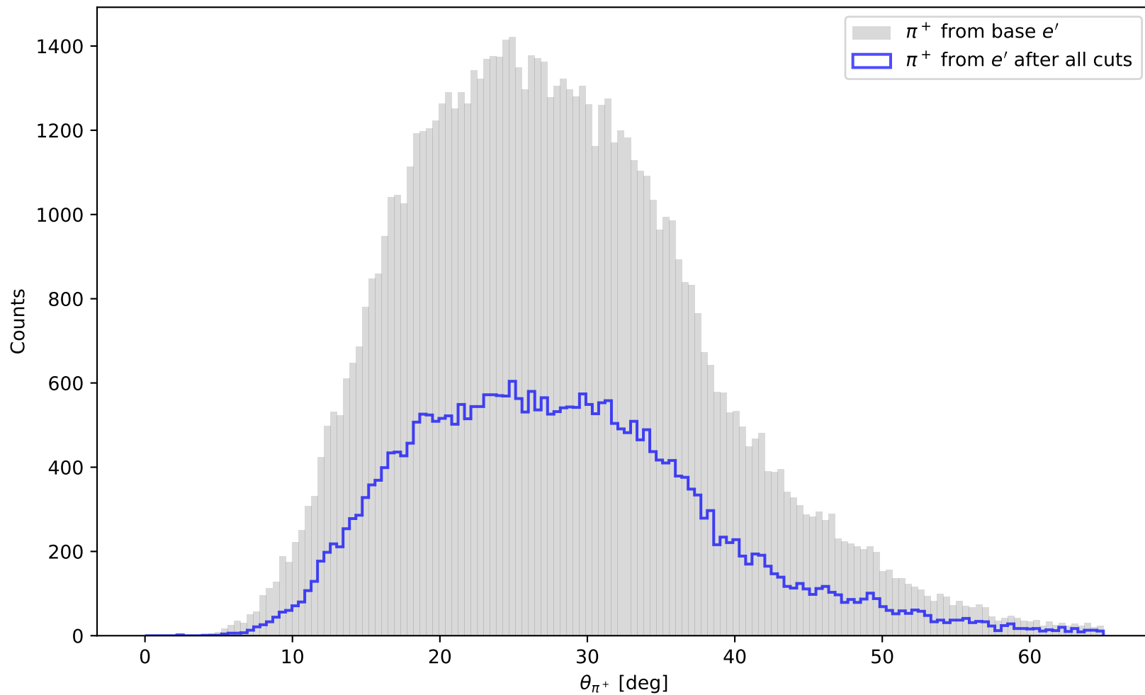
\theta_{\pi^+} Distribution
