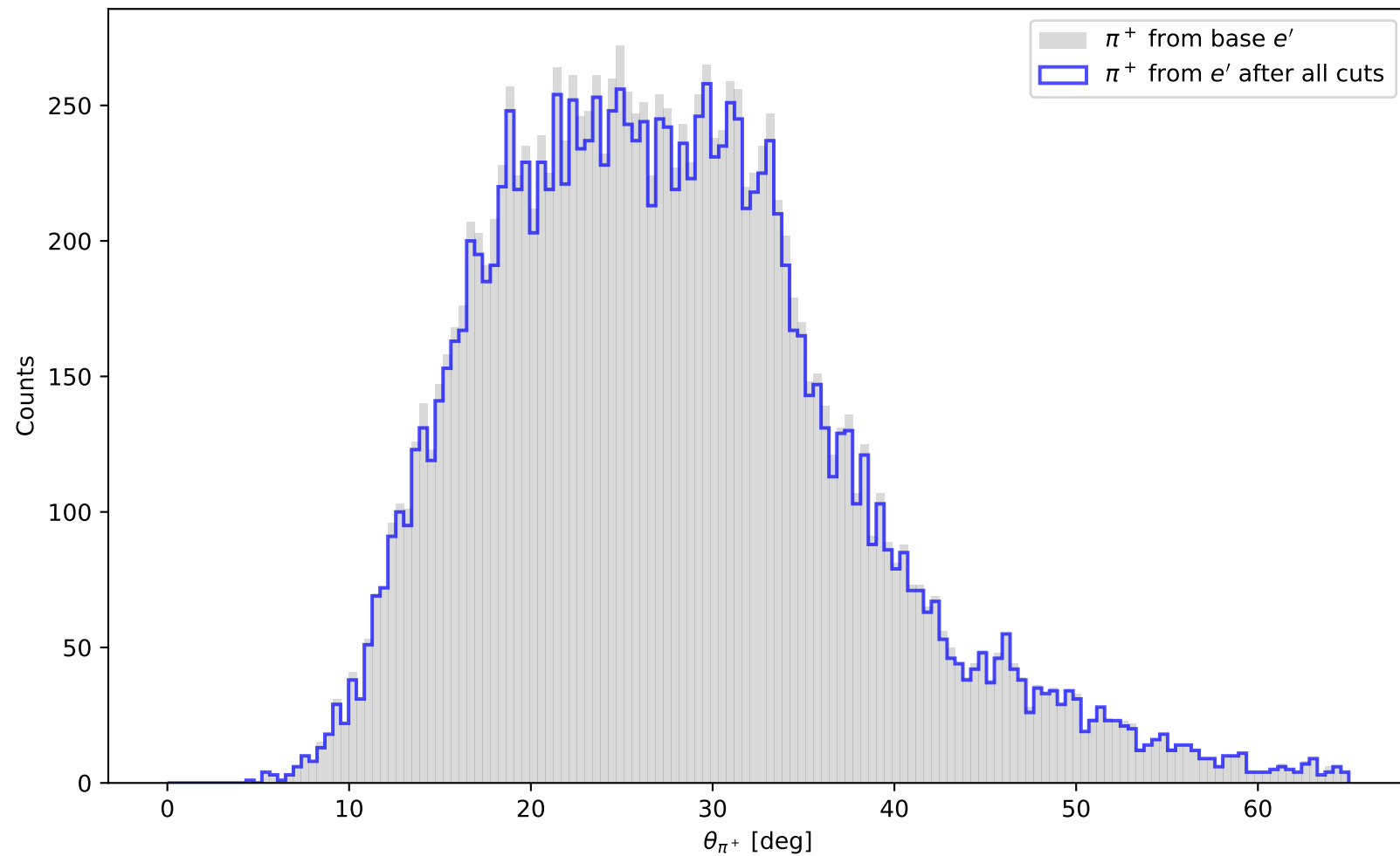
\theta_{\pi^+} Distribution
