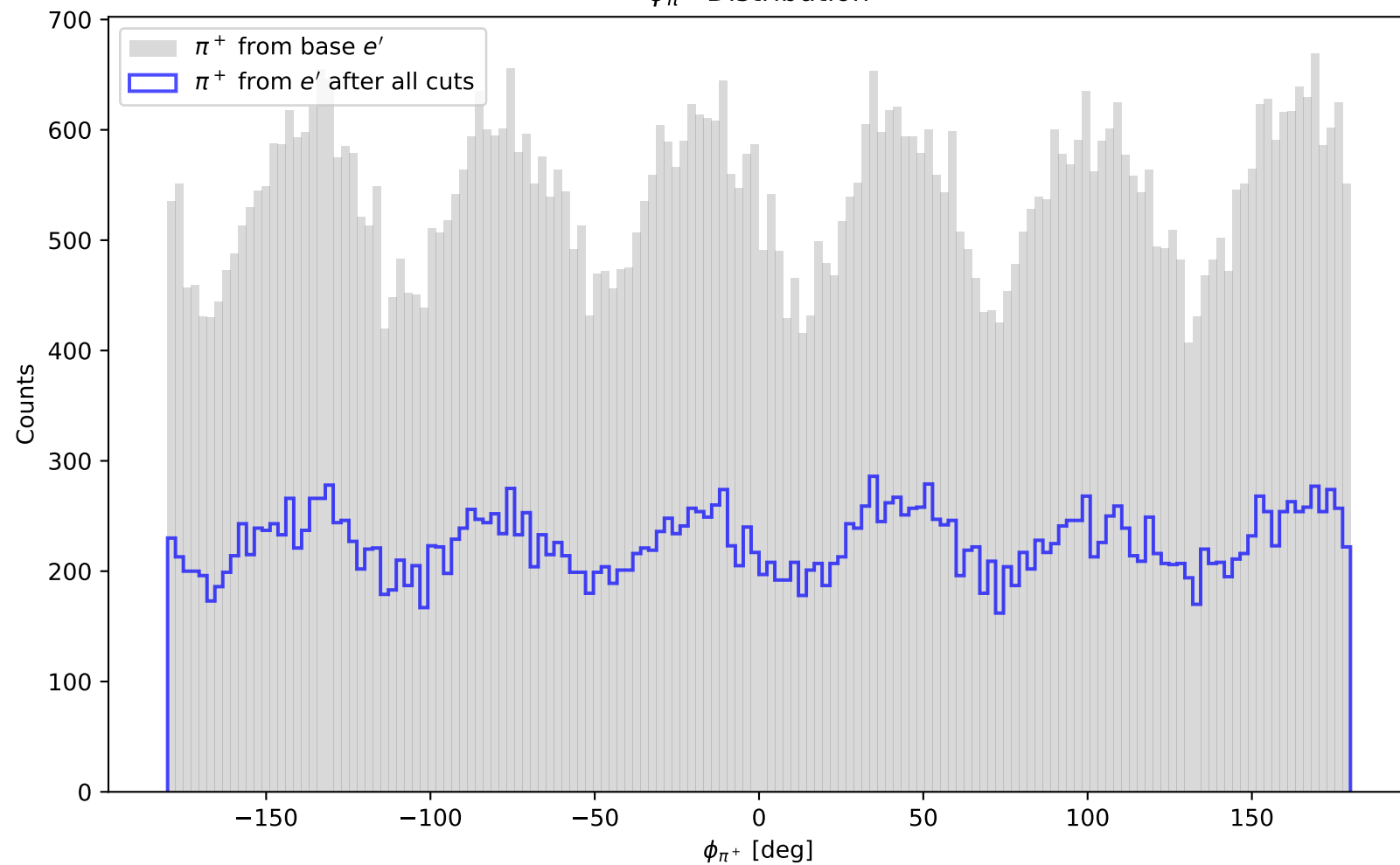
\phi_{\pi^+} Distribution
