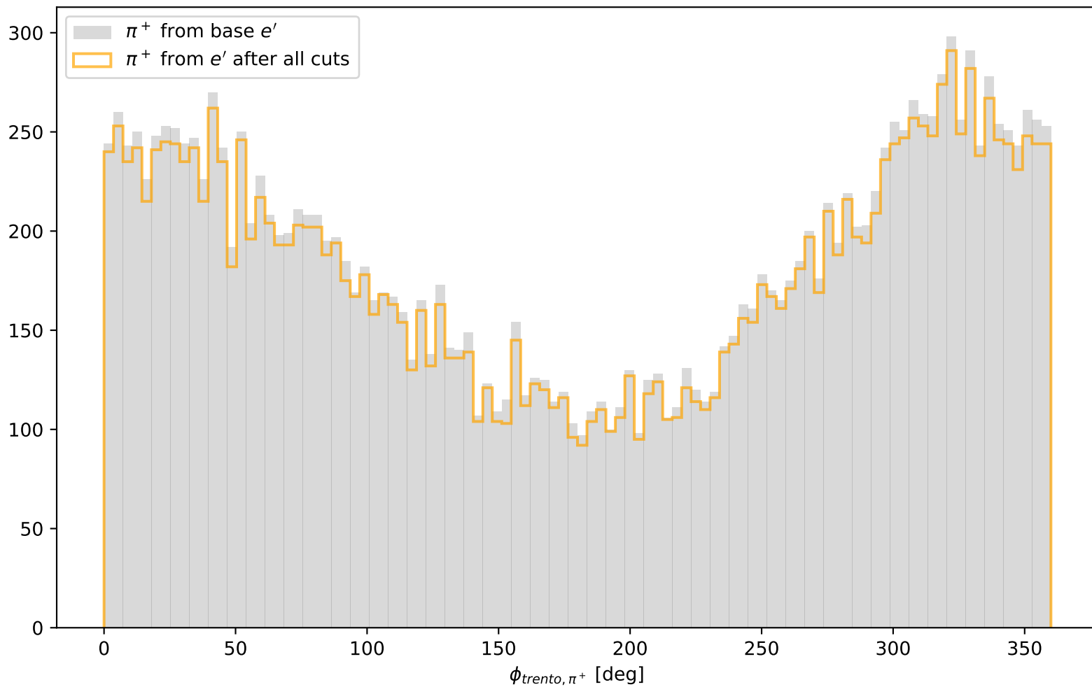
Trento Azimuthal Angle \phi_{trento,\pi^+}
