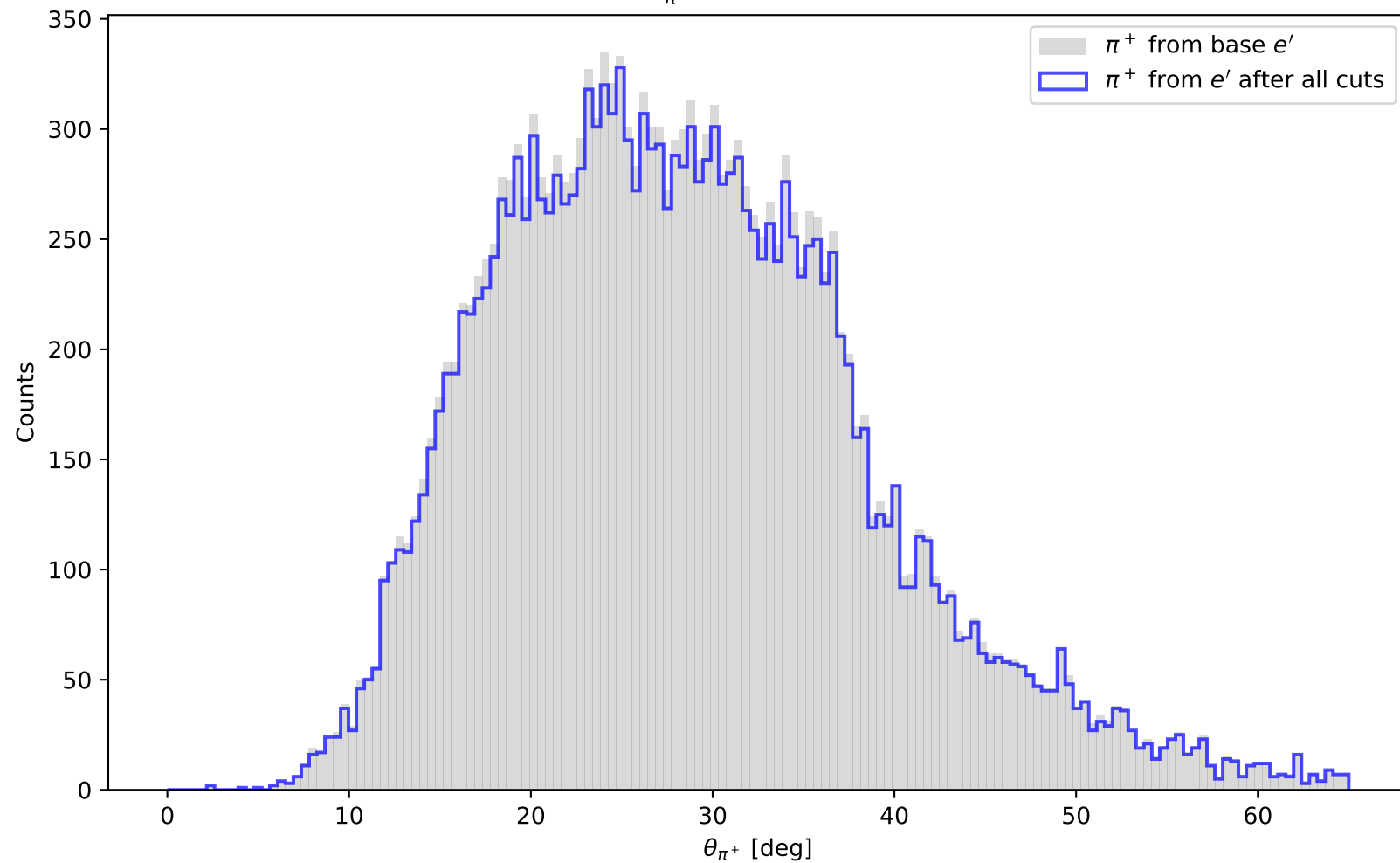
\theta_{\pi^+} Distribution
