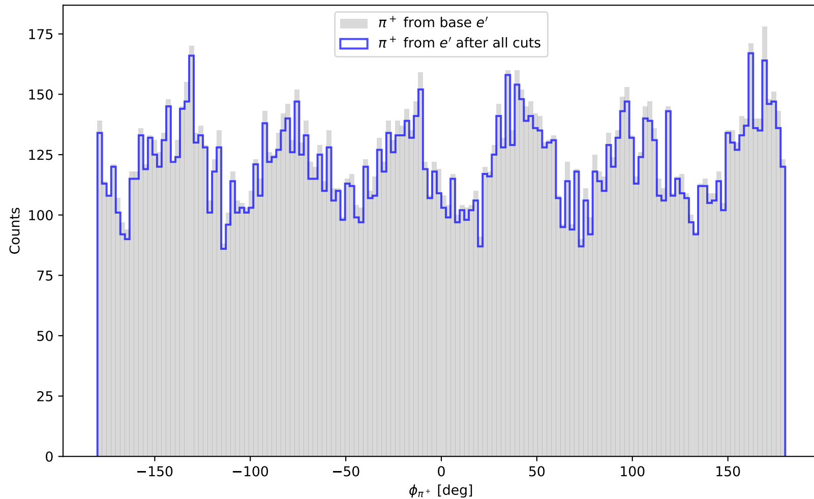
\phi_{\pi^+} Distribution
