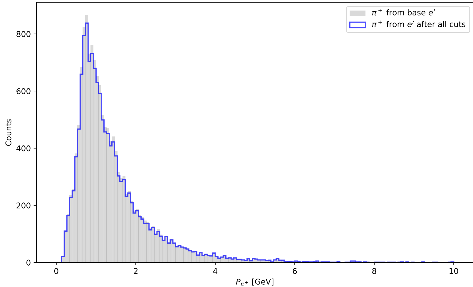
P_{\pi^+} Distribution
