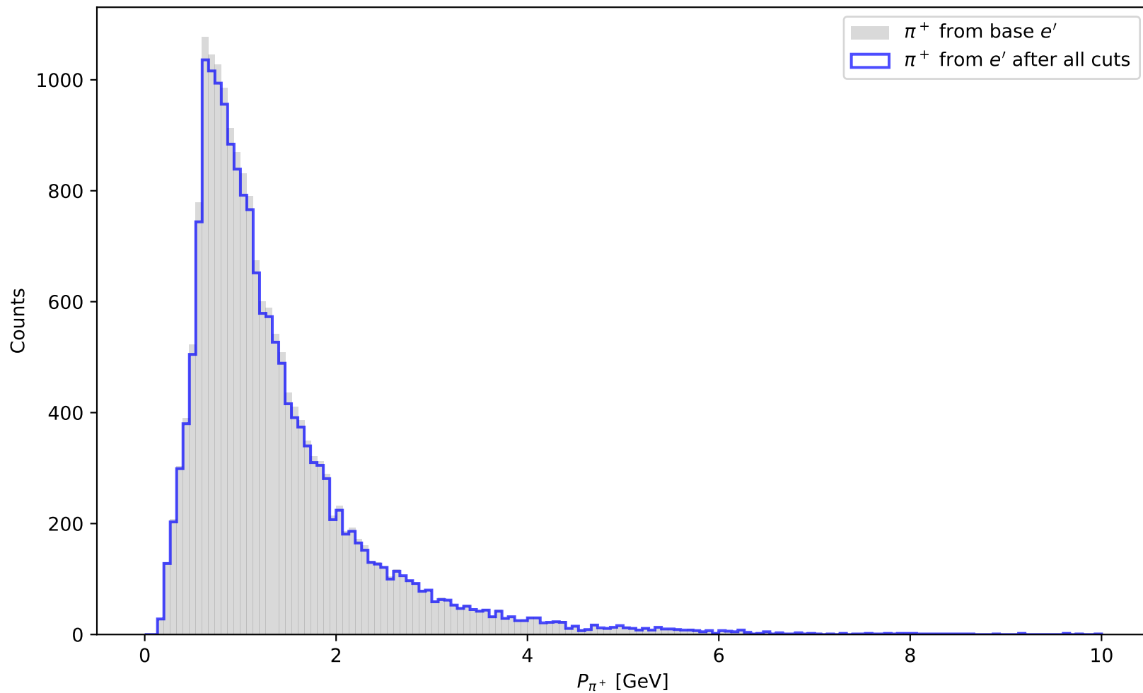
P_{\pi^+} Distribution
