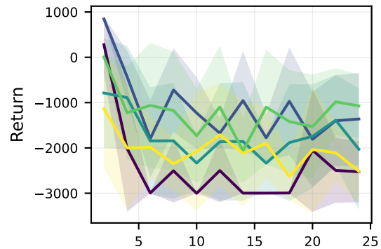
AntVelocity
