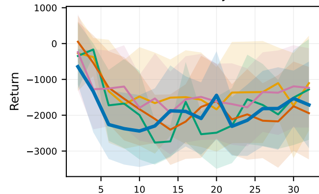
AntVelocity
