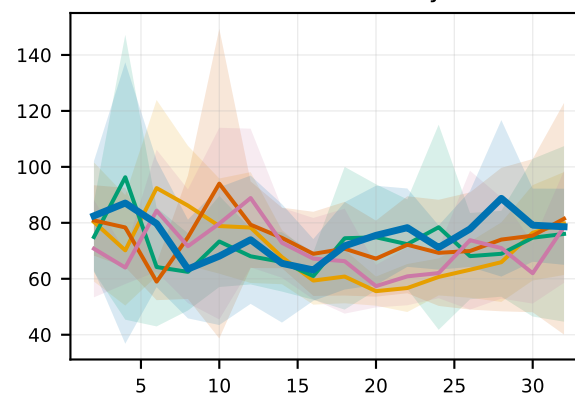
HumanoidVelocity
