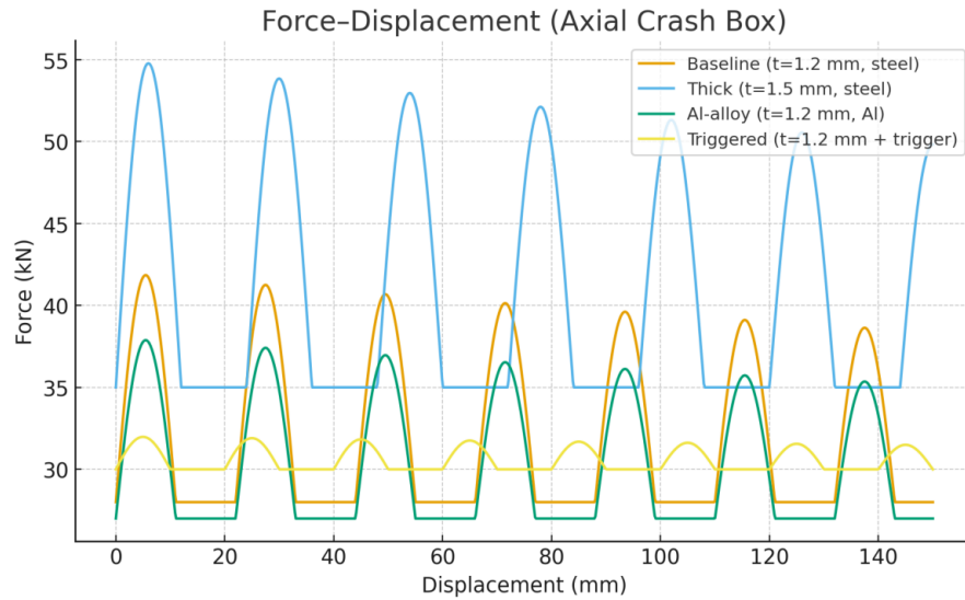
Force-Displacement
