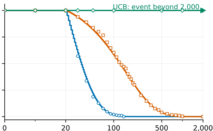
(d) Confirmed Q recovery; gap D = 1
