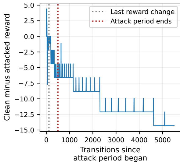
(d) Actual reward difference
