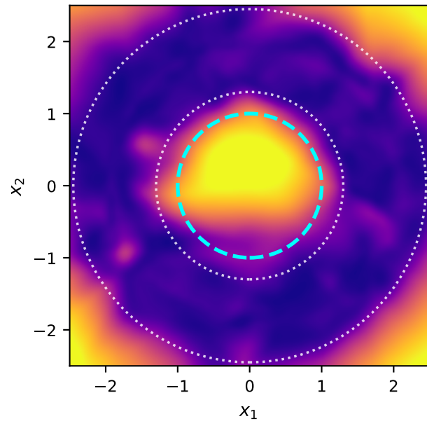
D. DP-BNN (Ours)
