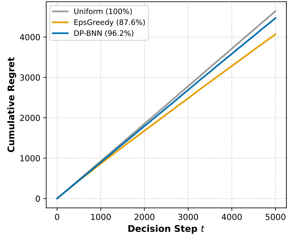
(d) Adult Census ( d = 93, K = 14 )
