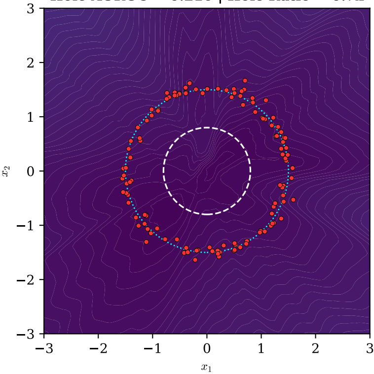
(d) Variational Inference Hole AUROC = 0.210 | Hole Ratio = 0.7x
