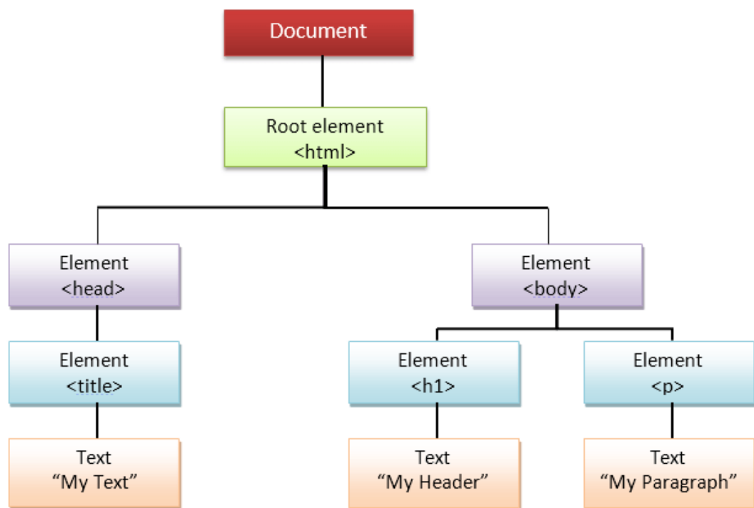
DOM Tree(Real)
