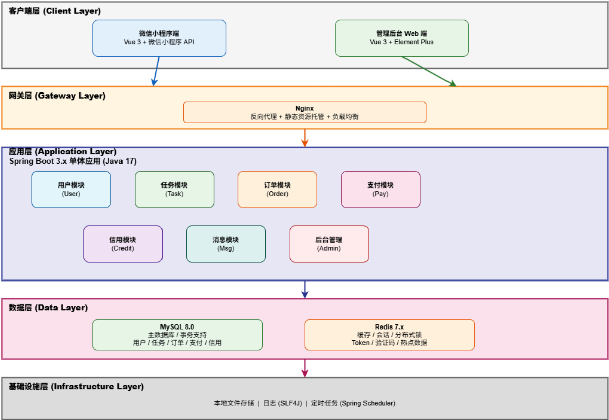
Campus Helper 系统架构图
