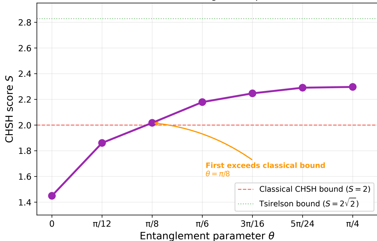
CHSH score vs entanglement parameter
