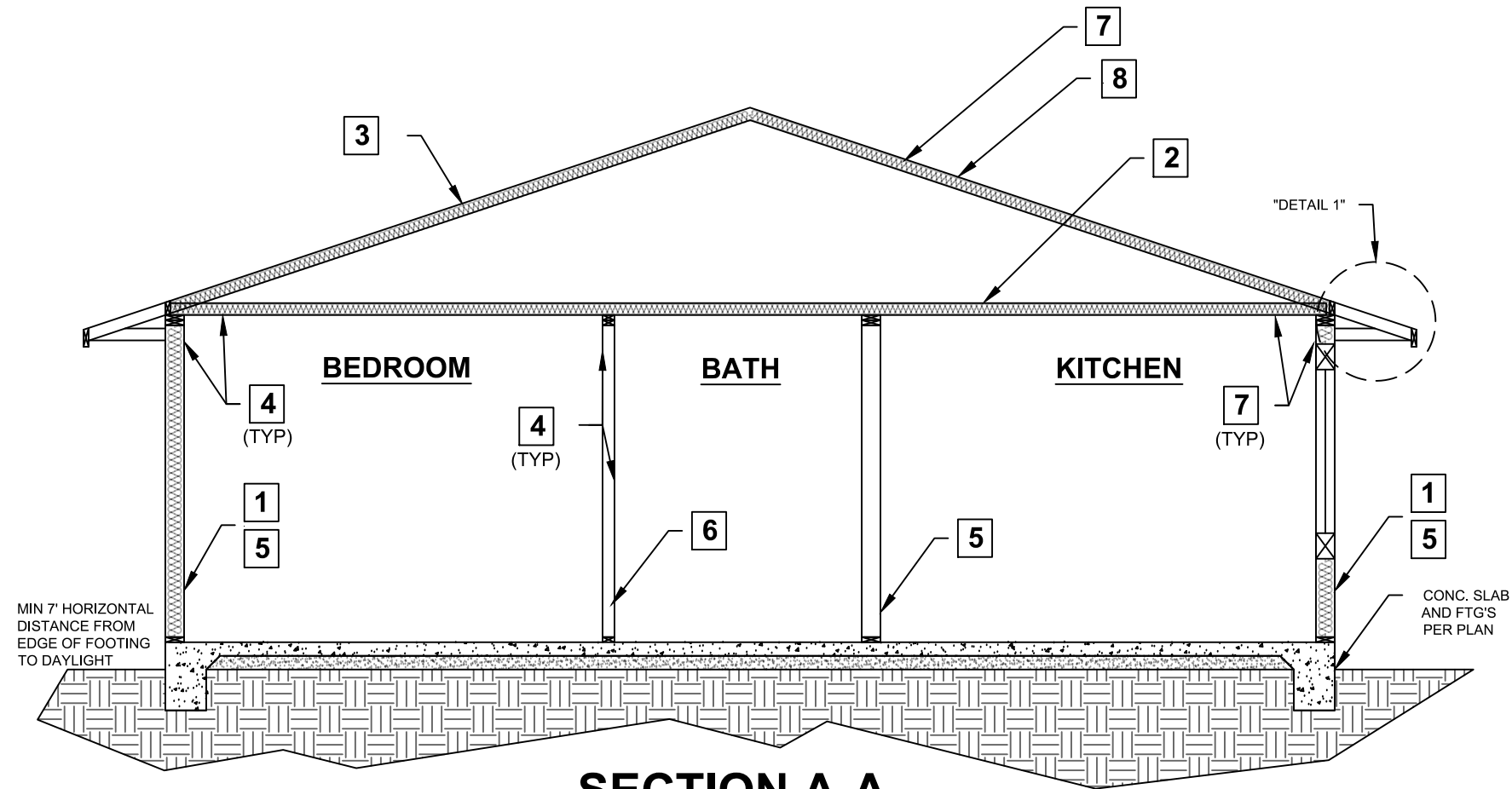
SECTION A-A
