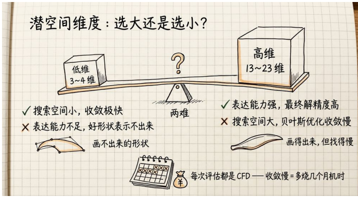
潜空间维度的两难：精度与收敛速率的冲突（latent dim dilemma，手绘笔记版）
