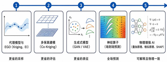
AI4Turbomachinery 技术演进路线图
