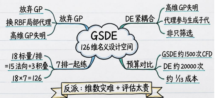
第03讲心智图：GSDE 高维 RBF 与 DE 紧耦合（mindmap）
