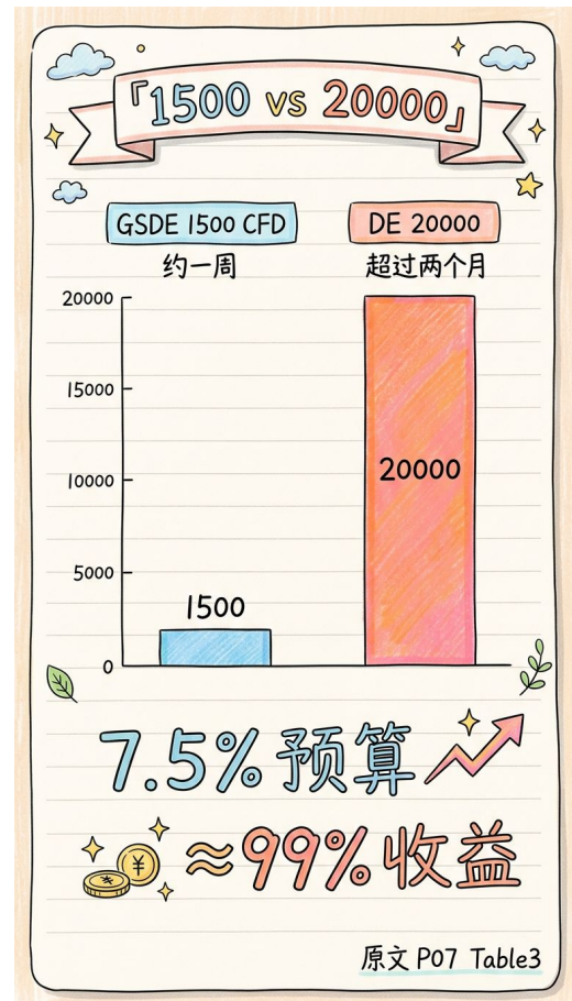
budget 1500 vs 20000: GSDE 与 DE 墙钟 [原文 P07 Table 3]
