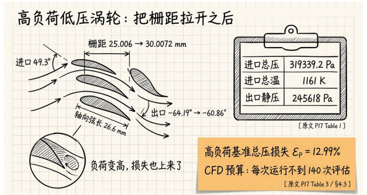
高负荷 LPT 叶栅几何与边界条件（blueprint points only，数值见 [原文 P17 Table 1]，手绘笔记版）
