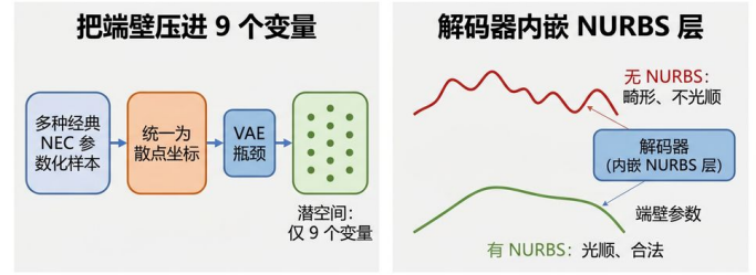
端壁生成式参数化与内嵌 NURBS 层 (VAE NURBS endwall, 中文标注版)
