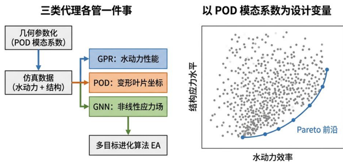
泵喷推进器流固耦合数字孪生流水线 (PJP digital twin, 中文标注版)
