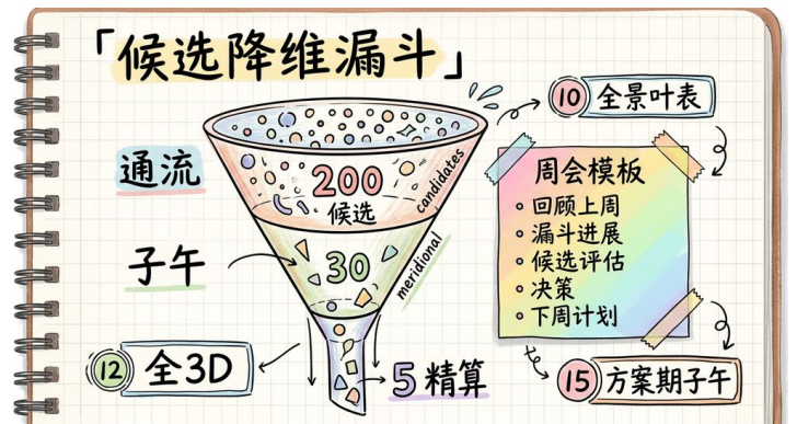
funnel wall: 通流200→子午30→全3D 5 的候选降维漏斗
