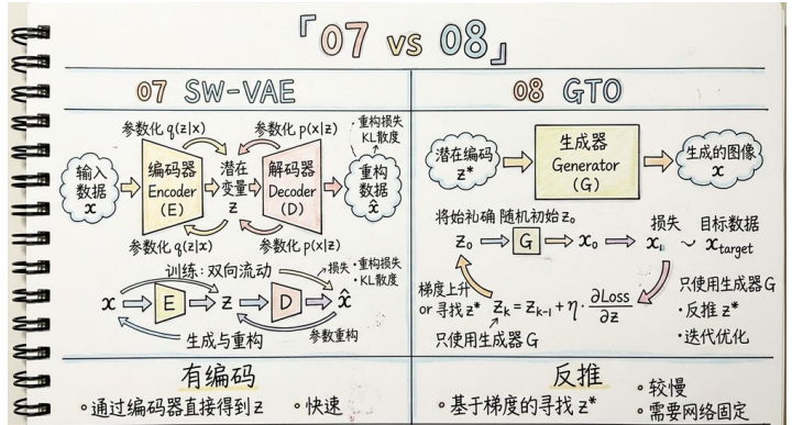
07 有编码器 vs 08 仅生成器+梯度反推
