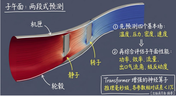
子午面流道与两段式预测框架（meridional two stage，概念渲染+手写批注版）
