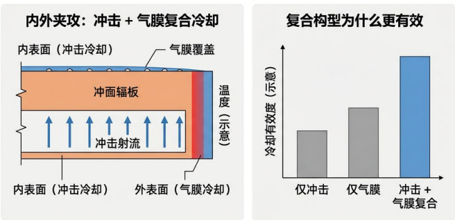
冲击加气膜复合冷却构型与效果对比 (impingement film cooling, 中文标注版)
