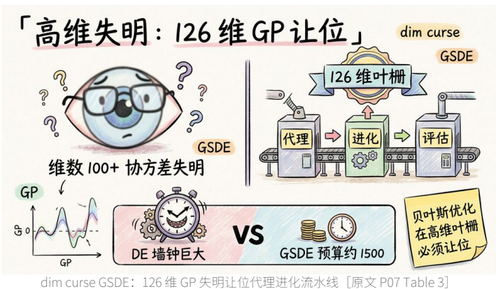
dim curse GSDE: 126 维 GP 失明让位代理进化流水线 [原文 P07 Table 3]
