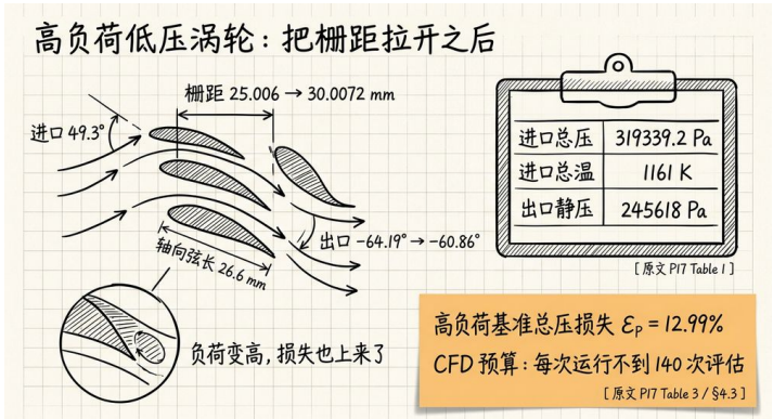
高负荷 LPT 叶栅几何与边界条件 (blueprint points only, 数值见 [原文 P17 Table 1], 手绘笔记版)
