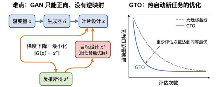
GAN 潜空间梯度反推与迁移热启动 (GTO gradient inversion, 中文标注版)
