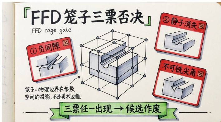
FFD cage gate 三票否决：负间隙 / 静子消失 / 不可铣尖角
