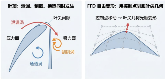
FFD 控制点网格与凹槽叶尖光顺变形 (ffd cage, 数值见 [出版商页面 摘要，论文 10]，手绘笔记版)
