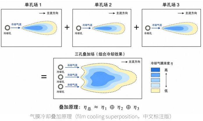
气膜冷却叠加原理（film cooling superposition，中文标注版）
