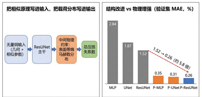
相似原理输入与物理增强收益对比（P-ResUNet similarity physics，中文标注版）
