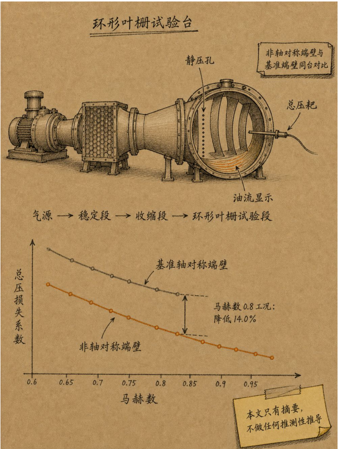
环形叶栅试验台流程与马赫数 0.8 工况降损 14.0% (cascade rig, 数值见 [原文 P09 摘要]，手绘笔记版)
