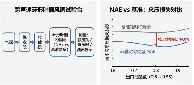
跨声速环形叶栅风洞试验台与损失对比 (transonic cascade windtunnel, 中文标注版)
