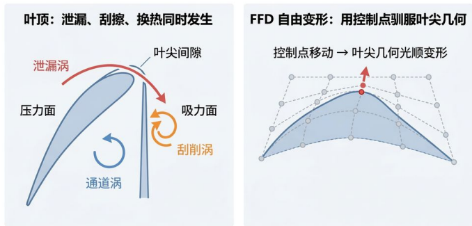
叶顶泄漏涡系与 FFD 控制点变形 (tip leakage FFD, 中文标注版) 上图是本讲全部内容的「一张图版本」：左图是叶顶为什么难——压力面到吸力面的泄漏流翻过叶尖间隙形成泄漏涡，与刮削涡、通道涡相互纠缠，同一块区域还承受着高热负荷；右图是 FFD 的解法——在叶尖表
