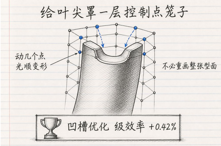
FFD 控制点网格与凹槽叶尖光顺变形 (ffd cage, 数值见 [出版商页面 摘要，论文 10]，手绘笔记版)
