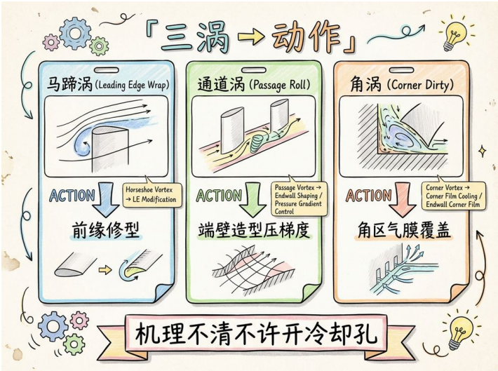
vortex to action: 马蹄/通道/角涡 → 前缘修型 · 压梯度 · 角区气膜
