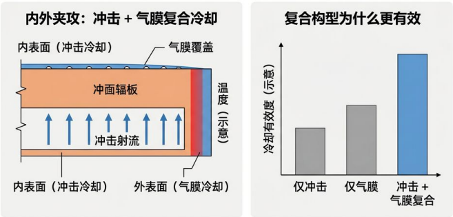
冲击加气膜复合冷却构型与效果对比 (impingement film cooling, 中文标注版)
