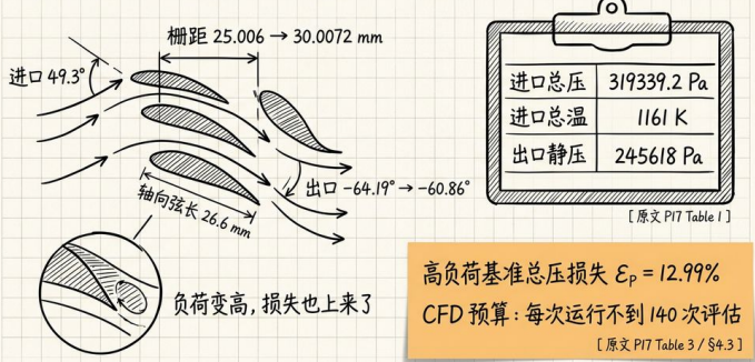
高负荷 LPT 叶栅几何与边界条件（blueprint points only，数值见 [原文 P17 Table 1]，手绘笔记版）
