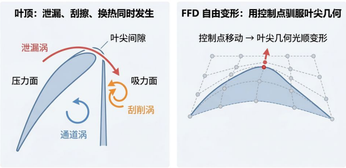
叶顶泄漏涡系与 FFD 控制点变形 (tip leakage FFD, 中文标注版)
