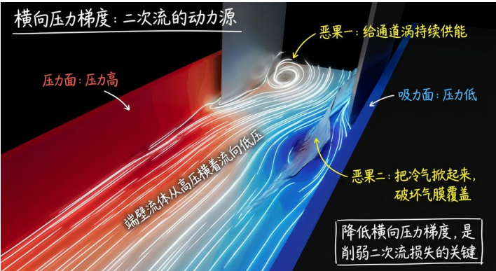
横向压力梯度驱动的端壁横向往及其两个恶果 (crossflow gradient, 概念渲染+手写批注版)
