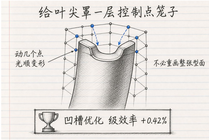
FFD 控制点网格与凹槽叶尖光滑变形 (ffd cage, 数值见 [出版商页面 摘要，论文 10]，手绘笔记版)
